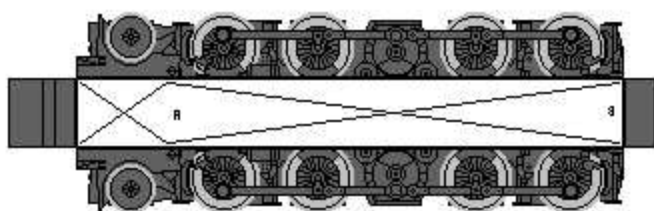
Malmtågslok litt Dm3 del 3
